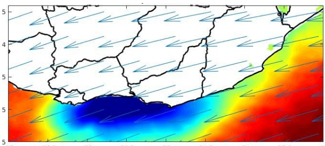
aSST GH NIÑA
