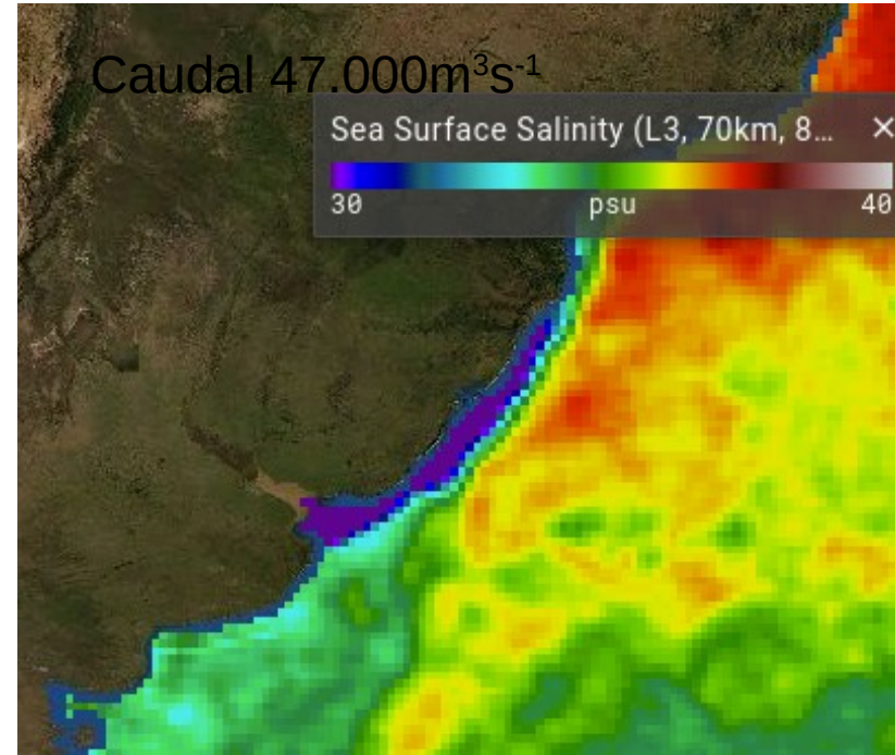
SMAP/REMSS 17/05/2016
