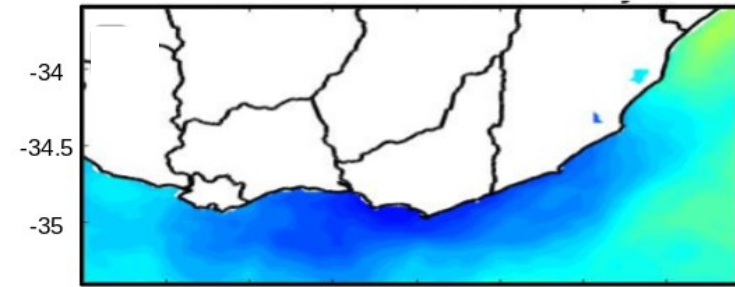
MUR-GHRRSST
