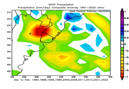
Menores precipitaciones → Menor descarga RdP
