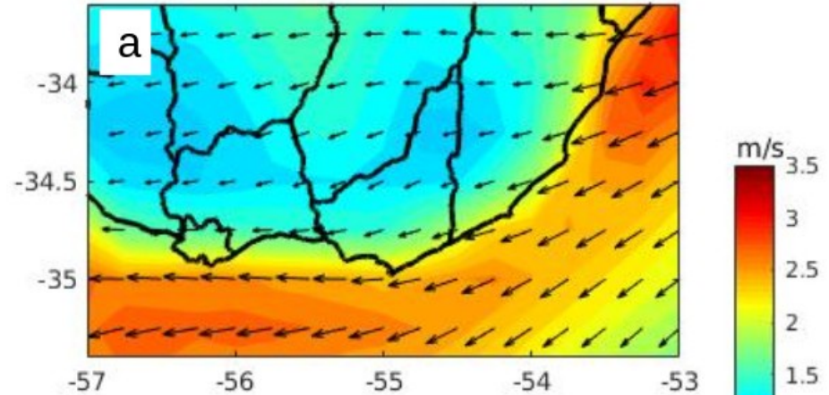
vientos medios JJA
