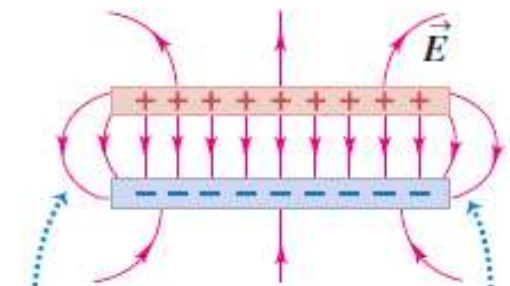
b) Vista lateral del campo eléctrico \vec{E}
