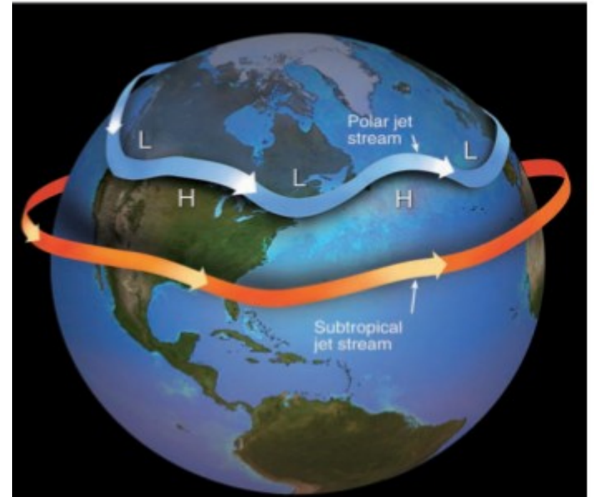
Jet streams polar (azul) y subtropical (naranja)
