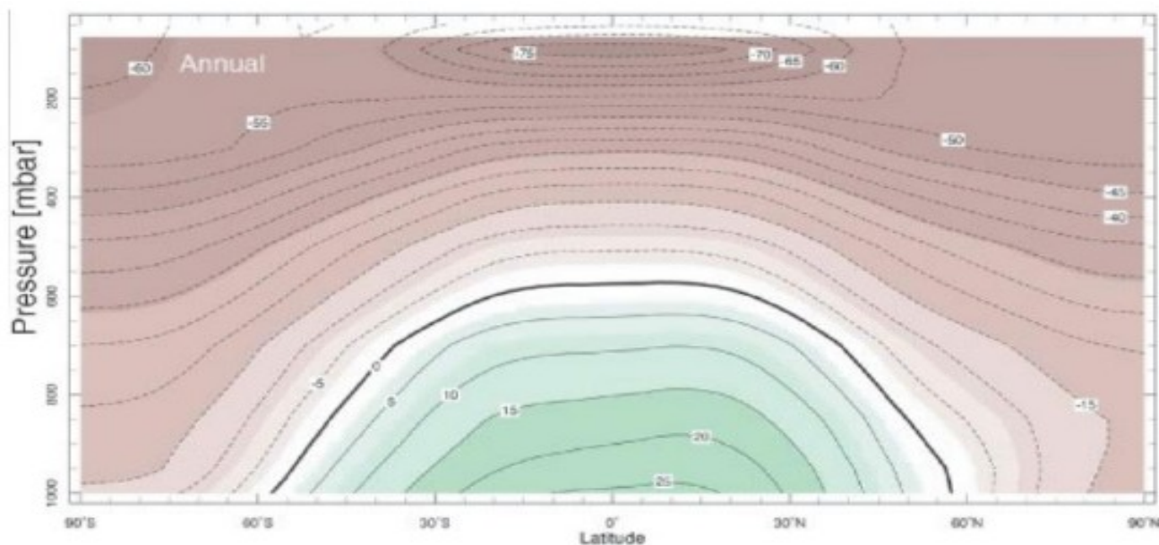
Temperatura promedio anual zonal de la atmósfera.
