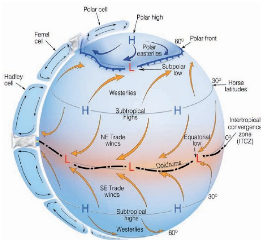
Modelo de tres celdas
